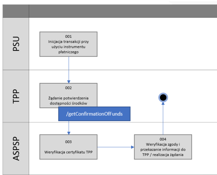
Ilustracja 18: CAF – zapytanie o dostępność środków
