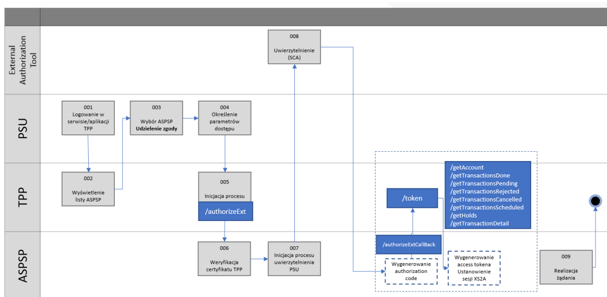
Ilustracja 12: AIS – ręczne wprowadzenie nr rachunku – uwierzytelnianie w zewnętrznym narzędziu autoryzacyjnym
