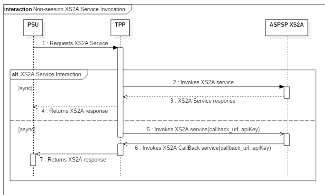
Ilustracja 29: Wywoływanie metod interfejsu XS2A bez użycia sesji
