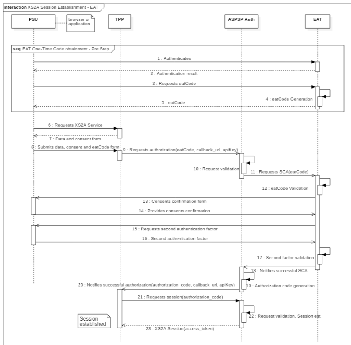
Ilustracja 25: Nawiązywanie sesji XS2A – metoda uwierzytelniania w zewnętrznym narzędziu autoryzacyjnym
