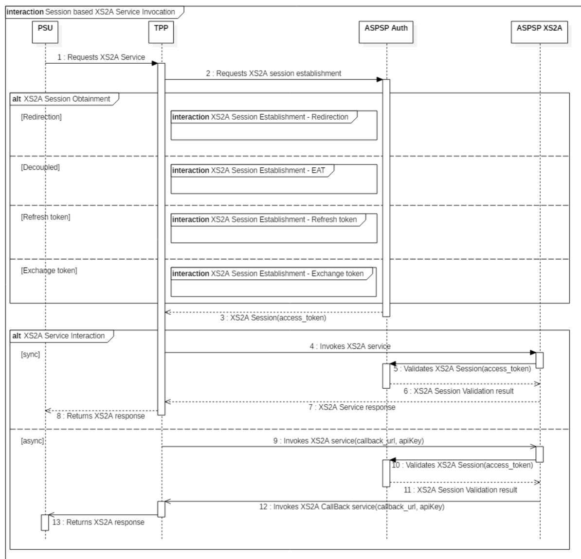
Ilustracja 28: Wywoływanie metod interfejsu XS2A z użyciem sesji
