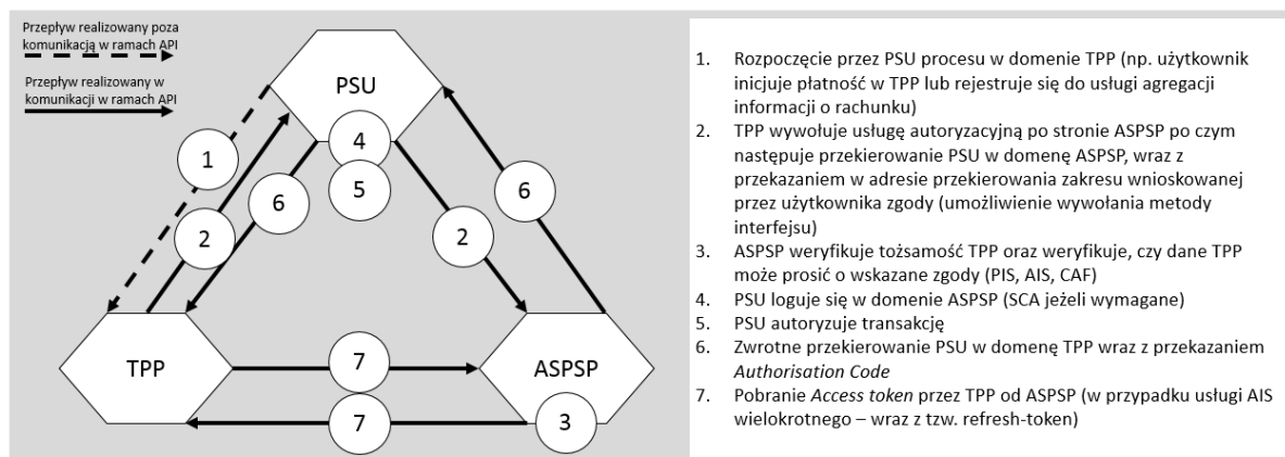
Ilustracja 20: Mechanizm uwierzytelniania po stronie ASPSP
