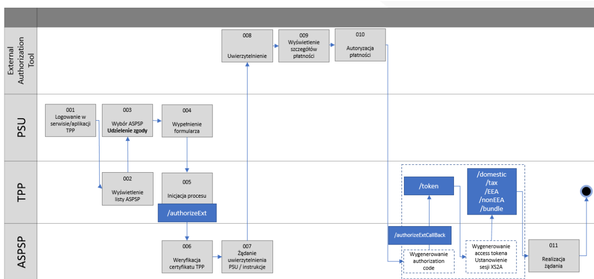
Ilustracja 6: PIS – uwierzytelnianie w zewnętrznym narzędziu autoryzacyjnym
